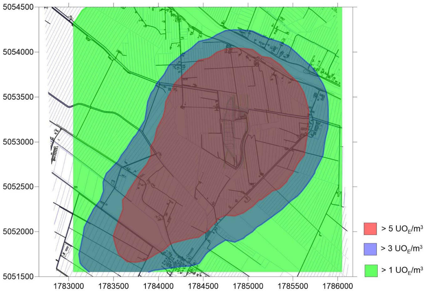
Figura 6 - Applicazione del modello di dispersione. Scenario Futuro. Concentrazione di odore relativo al 98esimo percentile (cfr. Linee guida Regione Lombardia)
