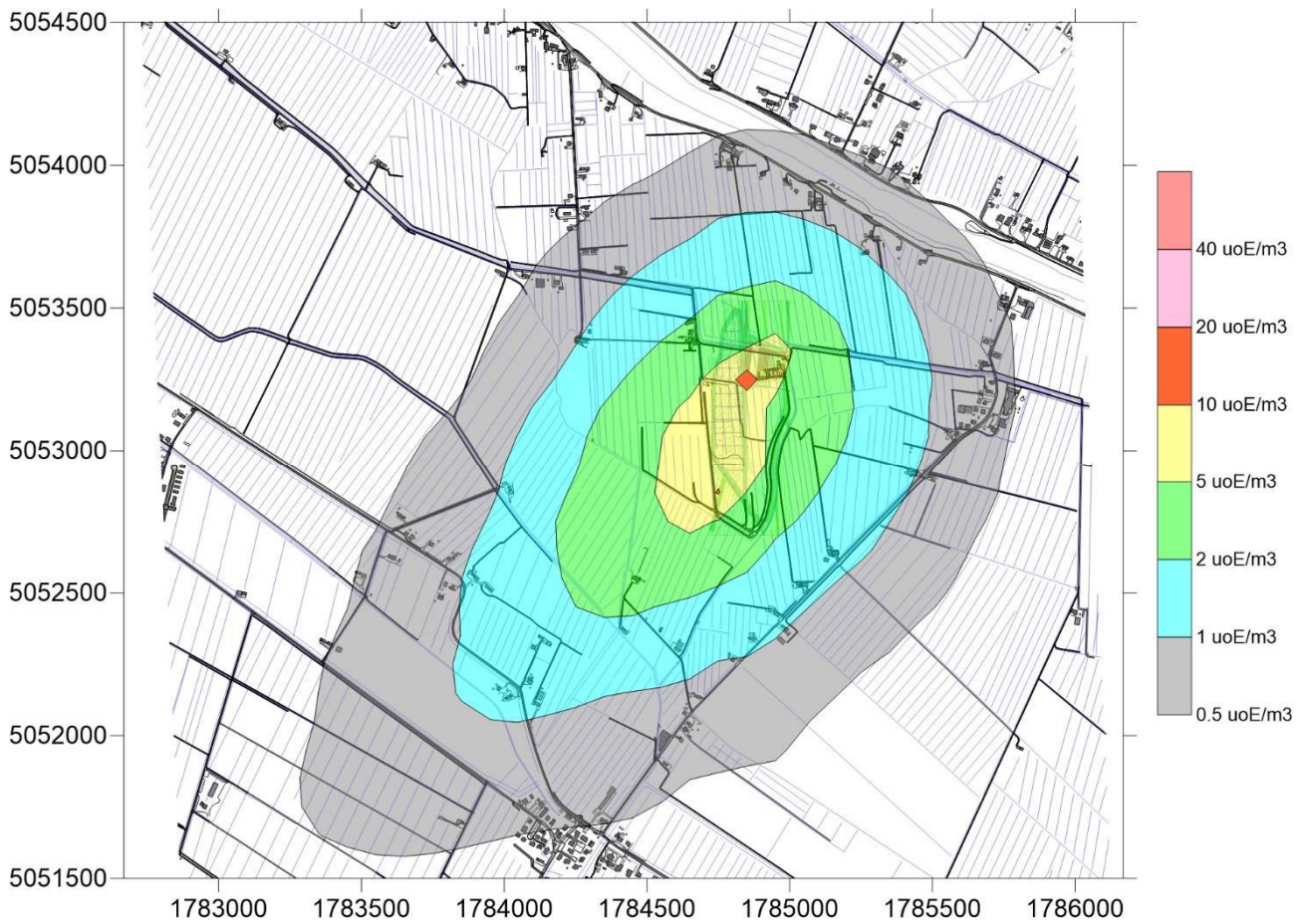
Figura 8 - Applicazione del modello di dispersione. Scenario Futuro. Concentrazione media di odore
