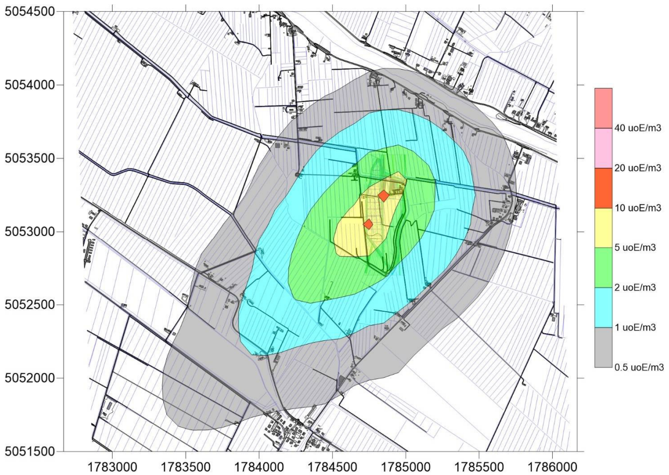
Figura 7 - Applicazione del modello di dispersione. Scenario Attuale. Concentrazione media di odore
